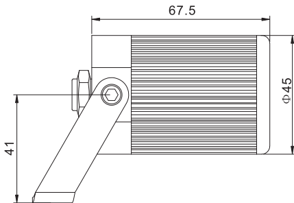
1 Montageloch D=7mm
