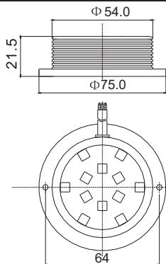
2 Montagelöcher D=5.0mm, Abstand 64mm
